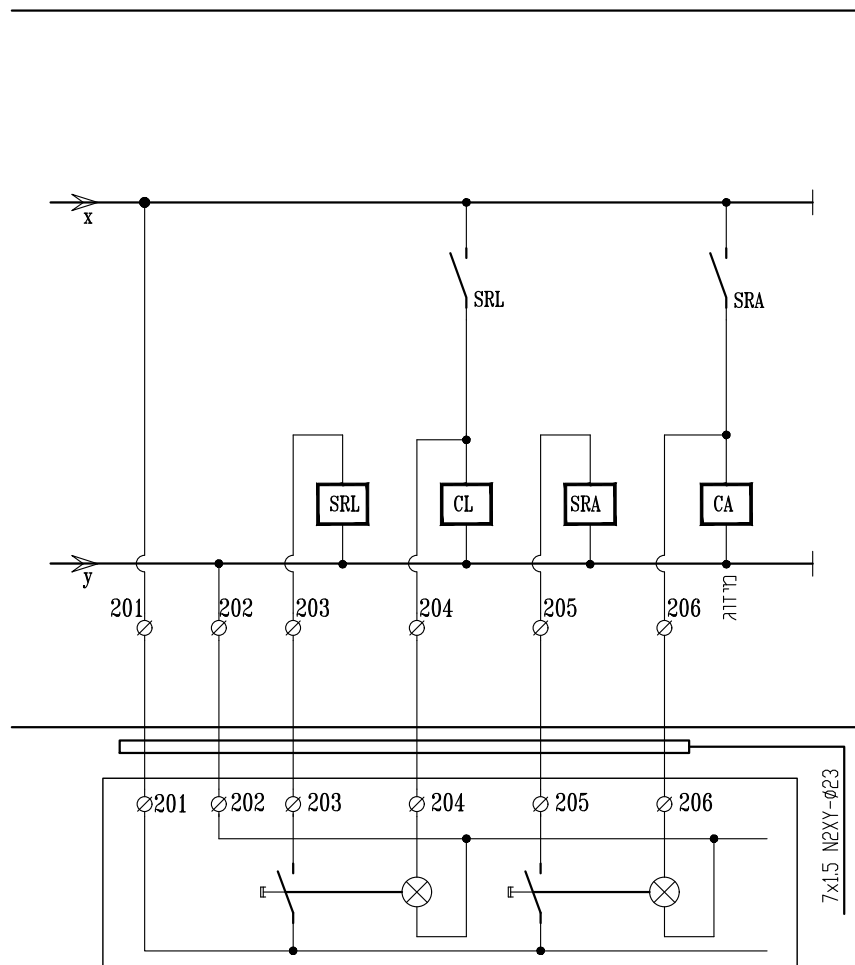
פנל כיבוי תאורה ומ.א. - 2 לחצנים מוארים
